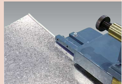
●片側で立上加工。
